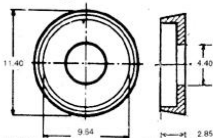
M201 (D) COMPONENT HOLDER DIODE CRADLE
